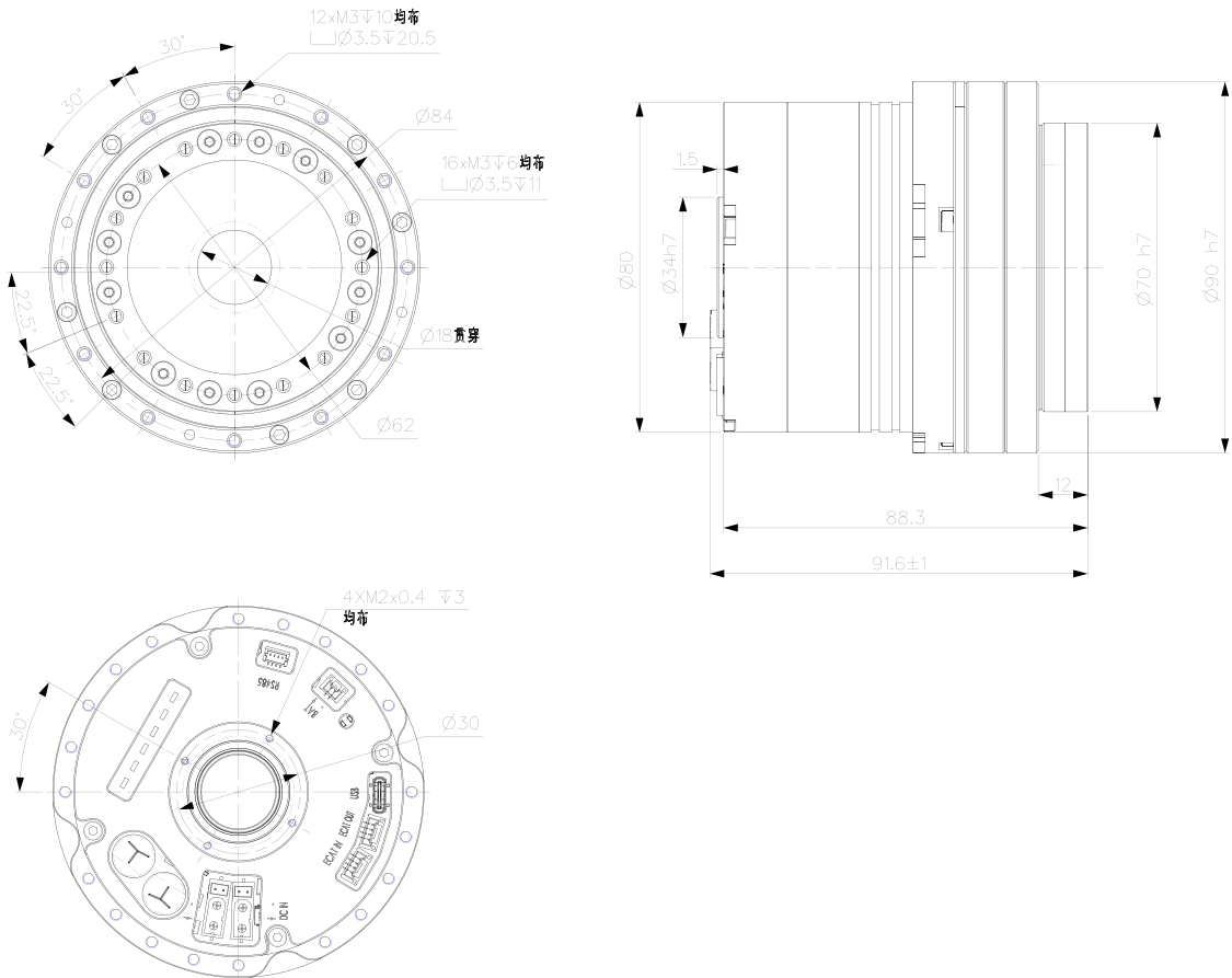
Dimensions
